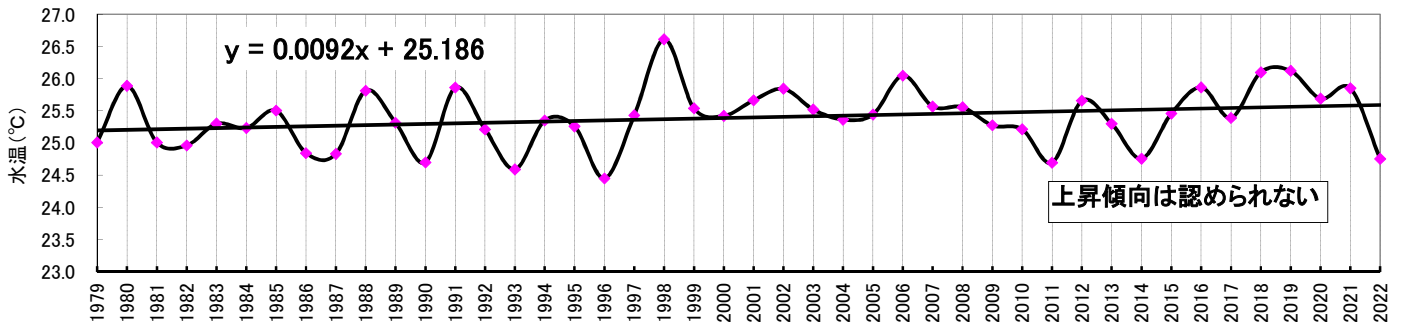
図 黒潮流域平均水温(4~6月)の推移
