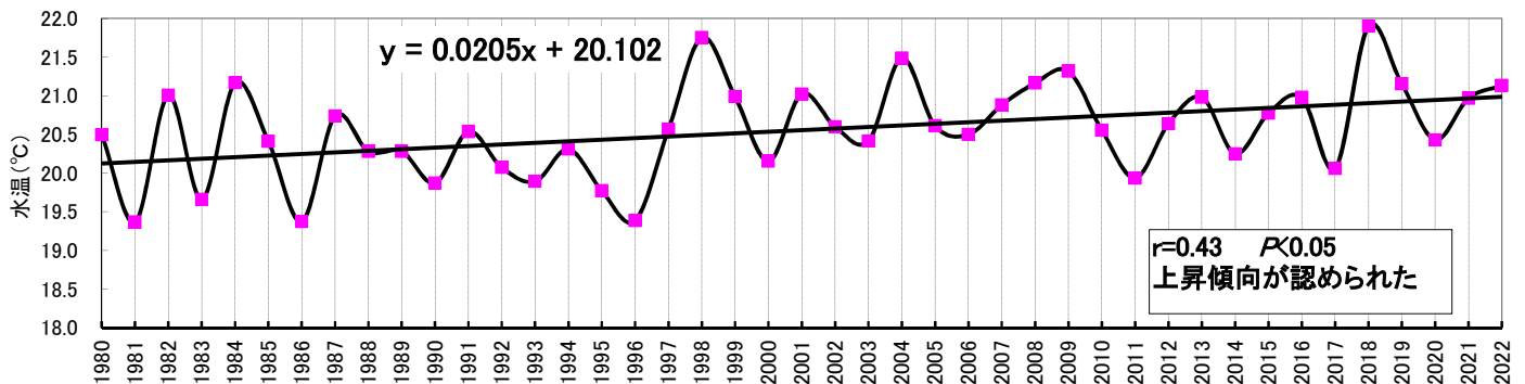
図 谷山平均水温(4~6月)の推移
