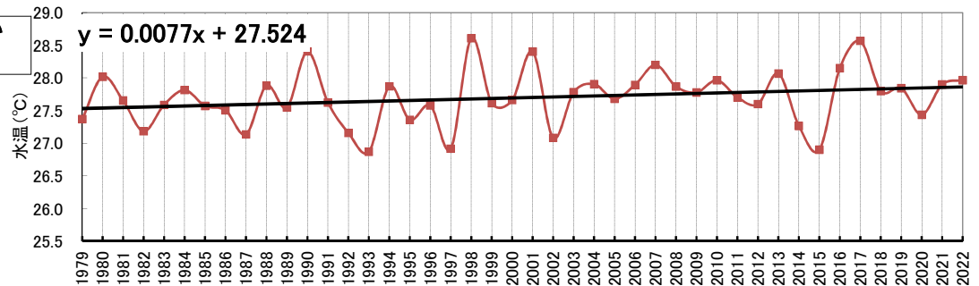
図 薩南沿岸平均水温（7～9月）の推移
