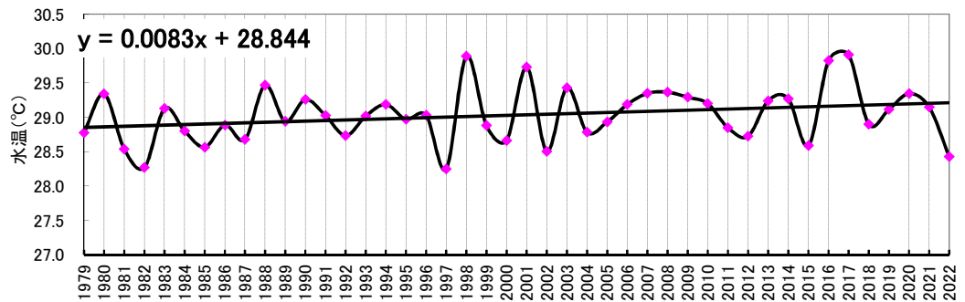
図 黒潮流域平均水温（7～9月）の推移
