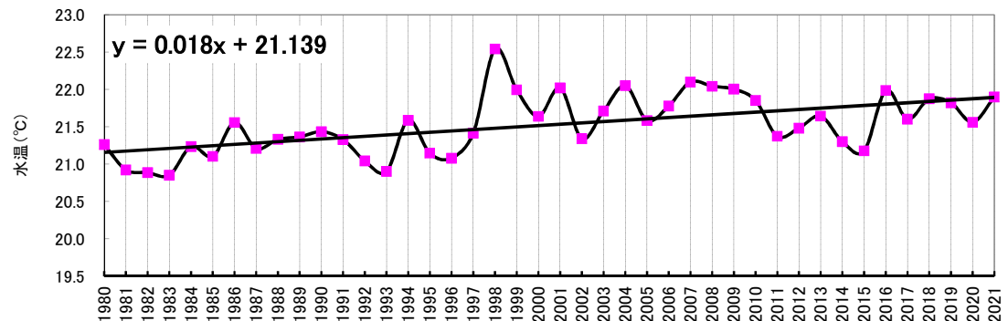
図 谷山年平均水温の推移
