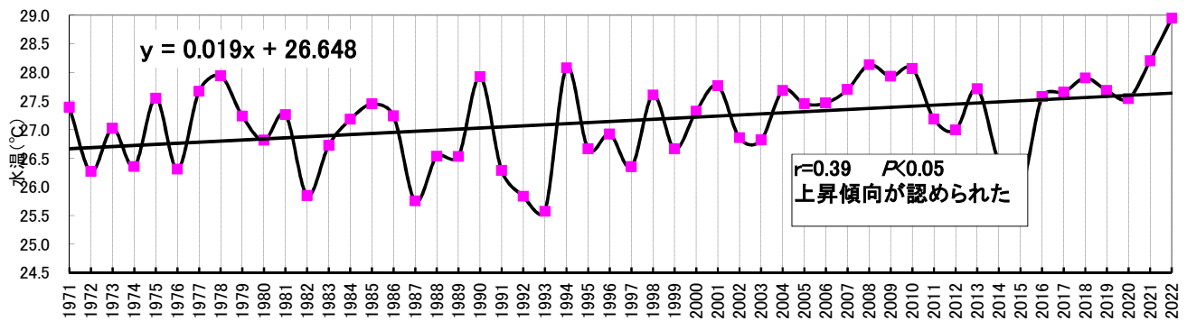
図 西薩沿岸平均水温（7～9月）の推移
