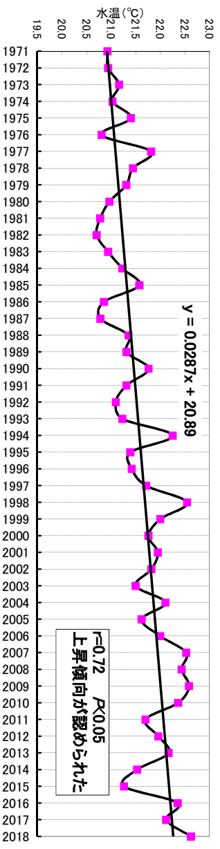
図 館海峽年平均水温の推移
