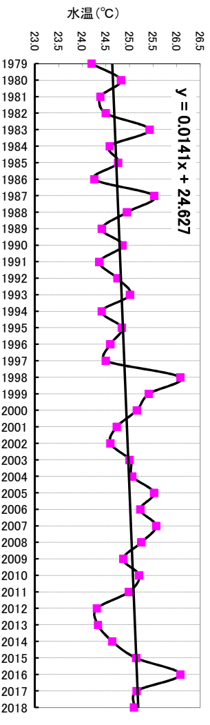
図 甕海峡平均水温（10～12月）の推移
