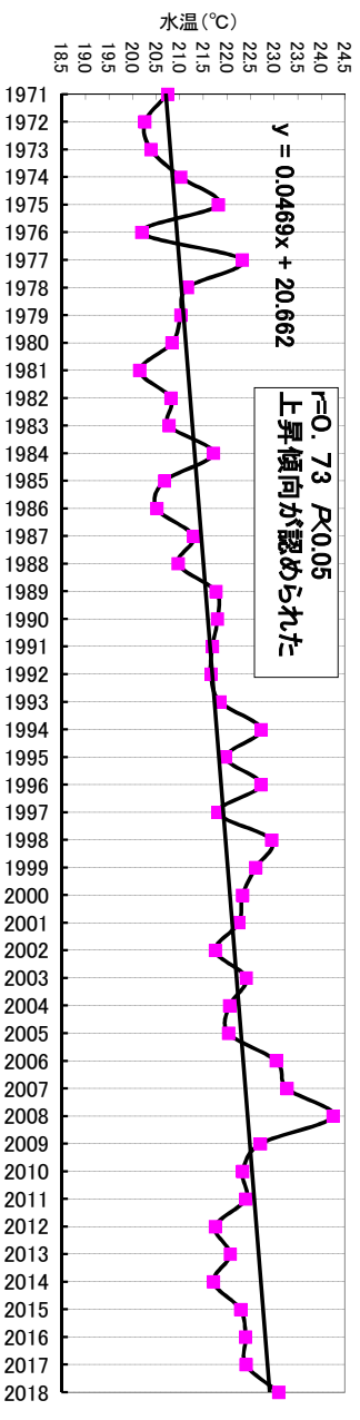
図 甕海峡平均水温（10～12月）の推移
