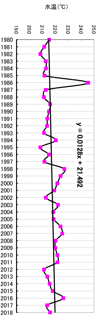
図 谷山平均水温（10～12月）の推移
