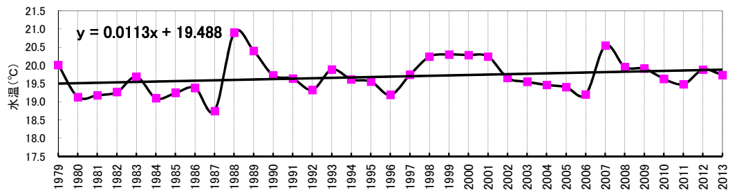
図 薩南沿岸年平均水温の推移
