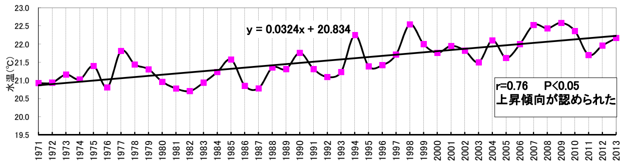
図 鰐海峡年平均水温の推移
