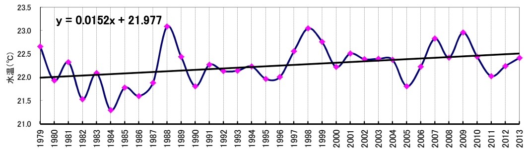
図 黒潮流域年平均水温の推移
