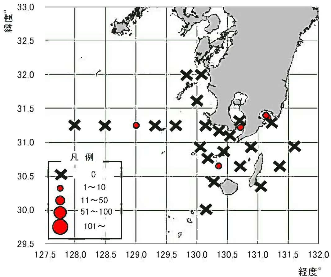
図 平成31年4月のウルメイワシ稚仔分布状況
