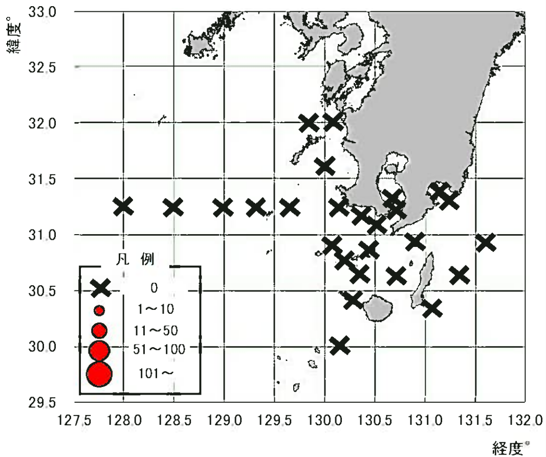
図 平成31年4月のマイワシ稚仔分布状況
