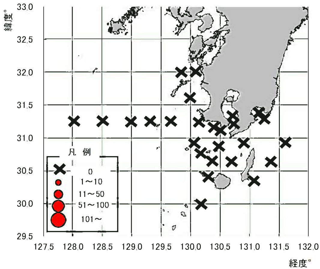
図 平成31年4月のマイワシ卵分布状況
