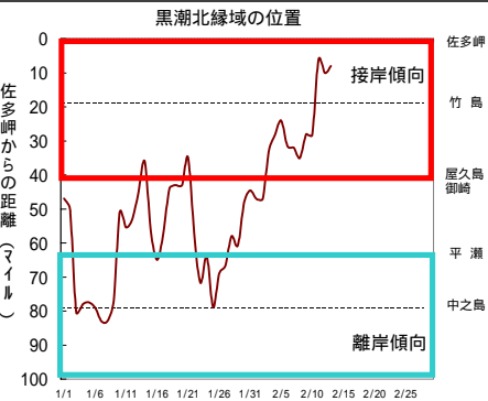
黒潮北縁域の位置
