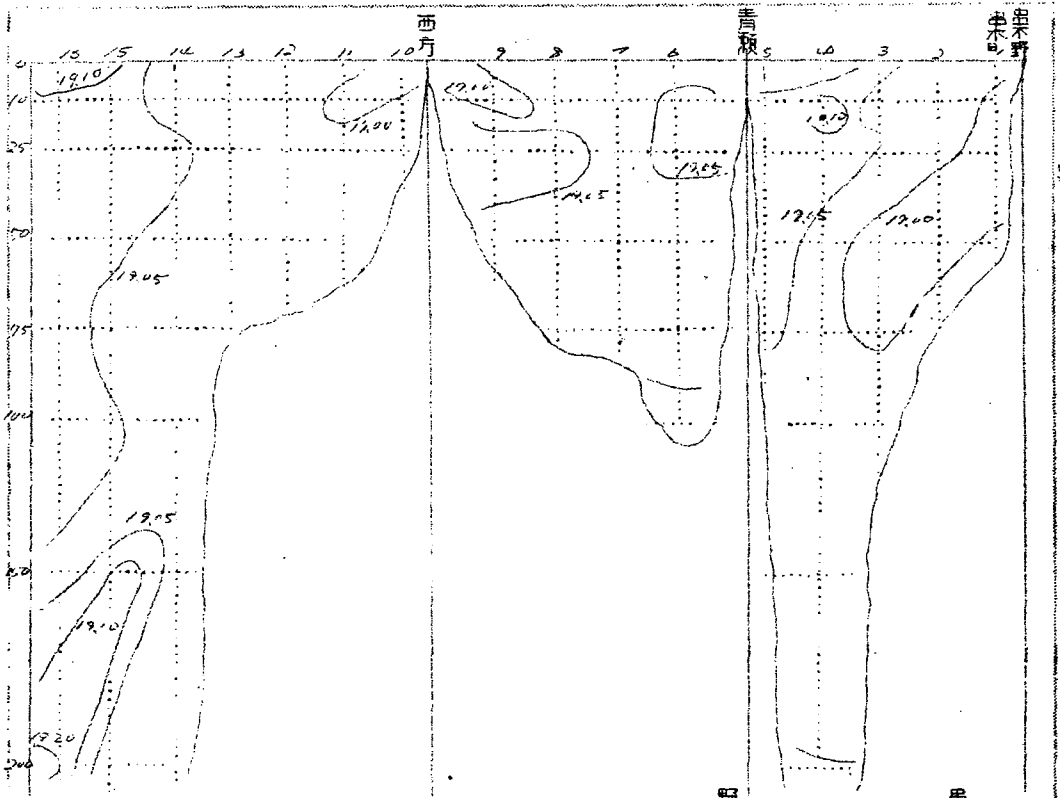
塩分鉛直断面分布図 (塩素量) % (十二月)
