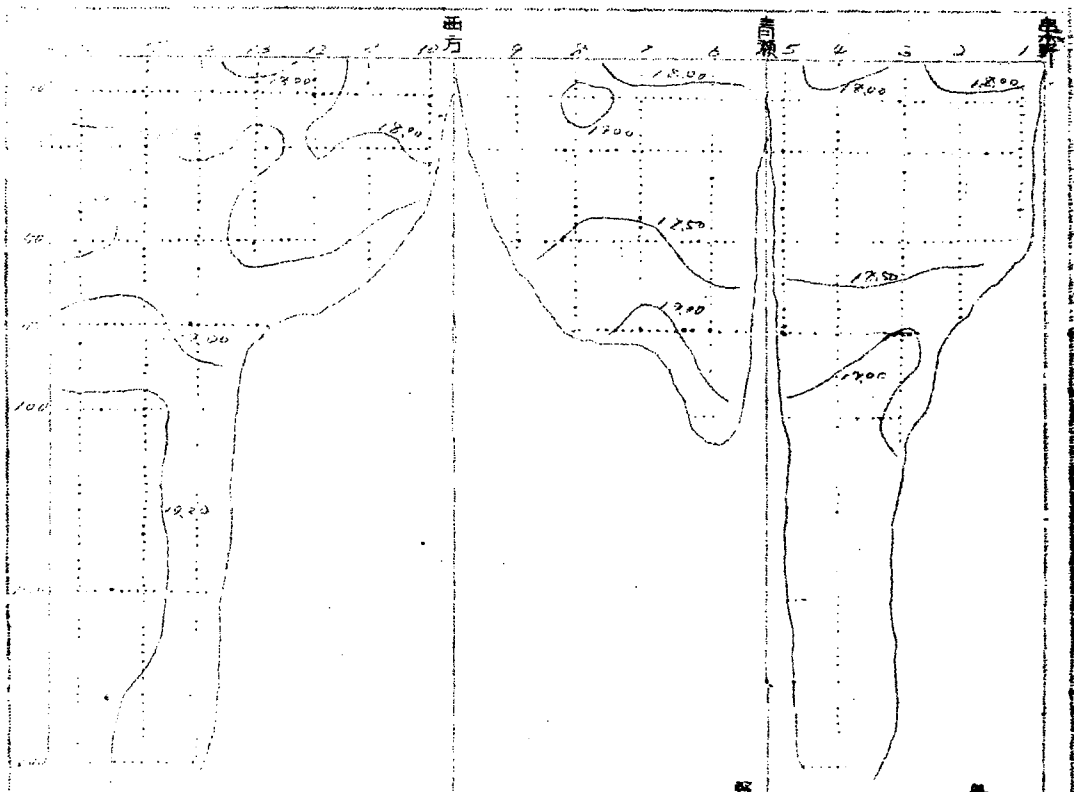
通分钻直断面分布图 (通泰堡) (八月)
