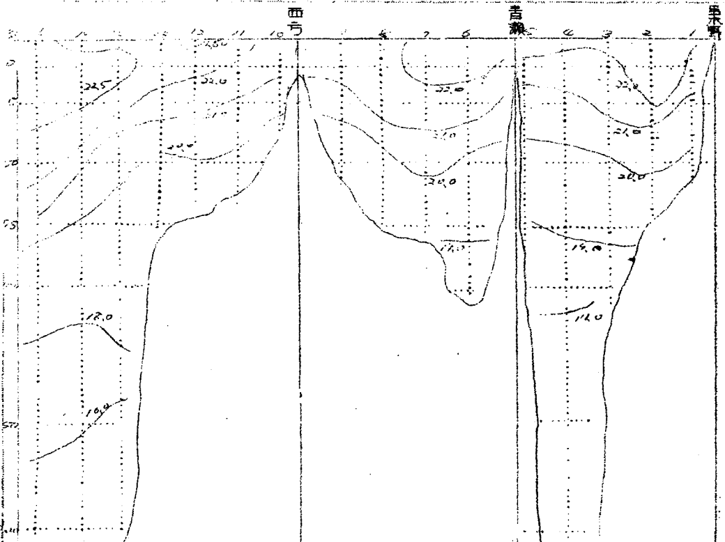
木温鉛直断面分布圖 ( ^{\circ}\text{C} ) (一二月)
