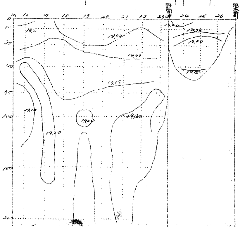
塩分鉛直断面分布図(塩分量)%(六月分)
