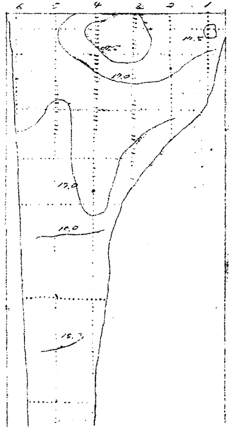
水温鉛直断面力布図 (四月) (°C)
