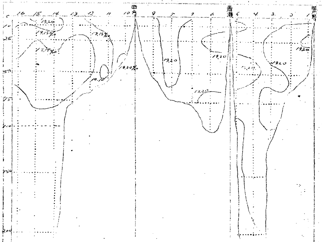
塩分飽和断面分布図(塩素量) % (二色)
