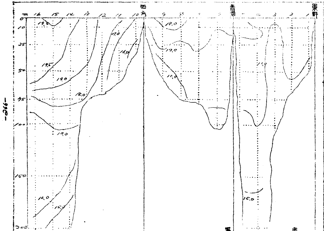
水温鉛直断面分布図 ( ^{\circ}\text{C} ) [三月]
