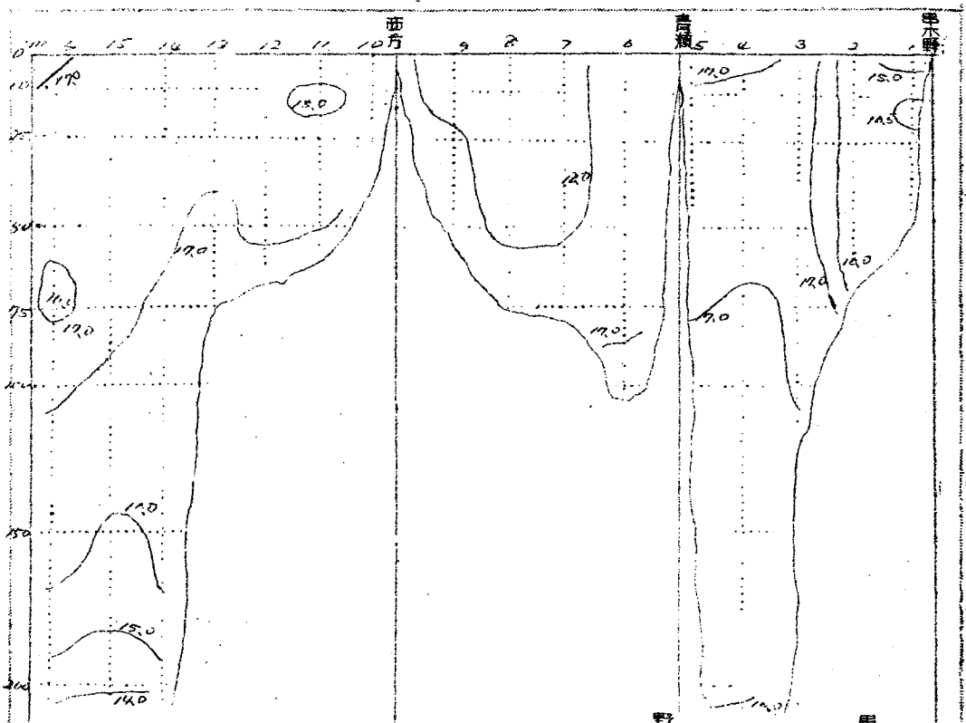
水温鉛直断面分布図 〔°C〕（二月）
