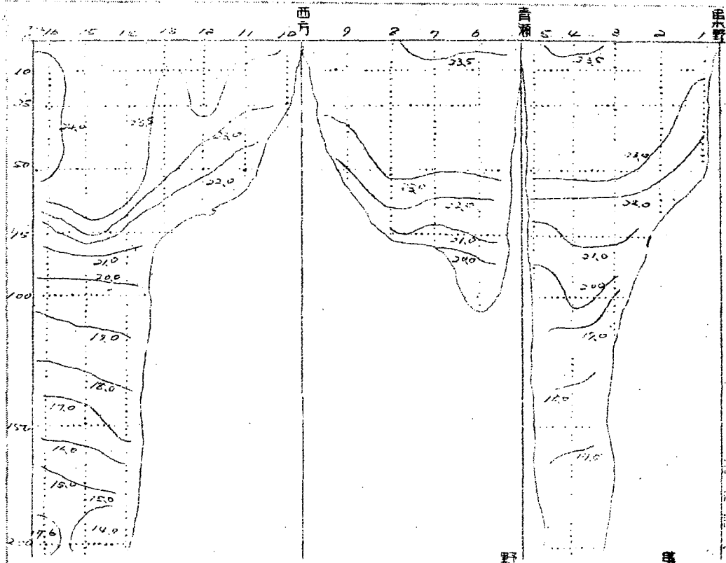
水温鉛直断面分布圖 〔C〕十一月
