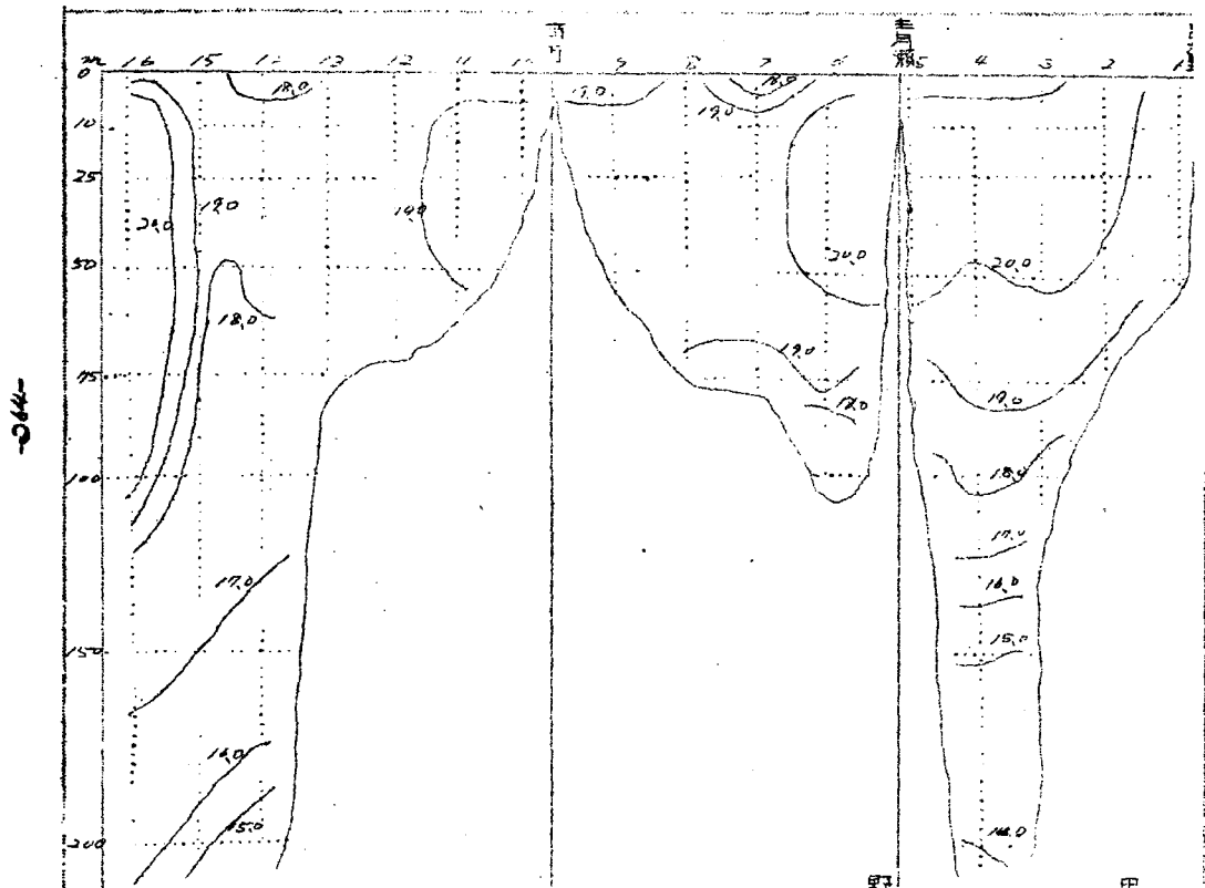
水温鉛直断面分布図 〔℃〕(二月)
