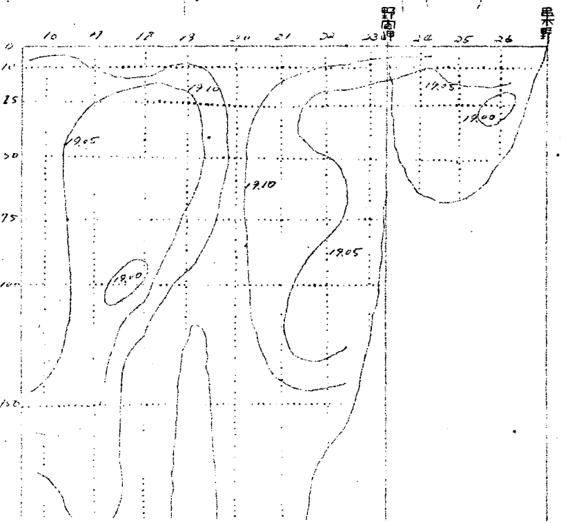
塩分鉛直断面分布図 (塩素量) % (十二月)
