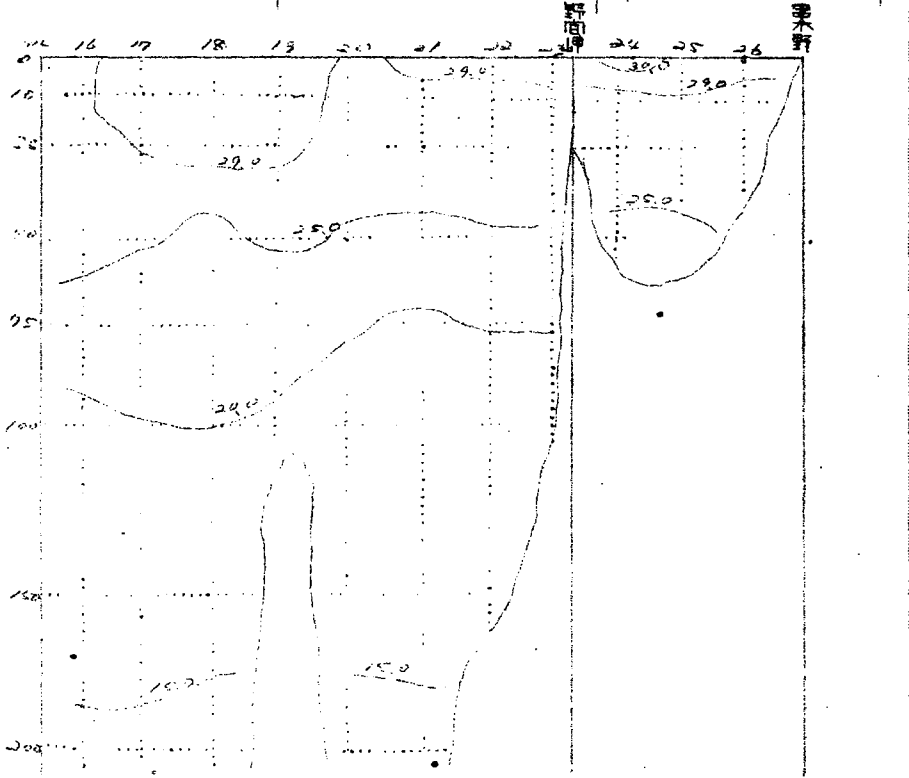
水温鉛直断面分布図 (°C) (八月)
