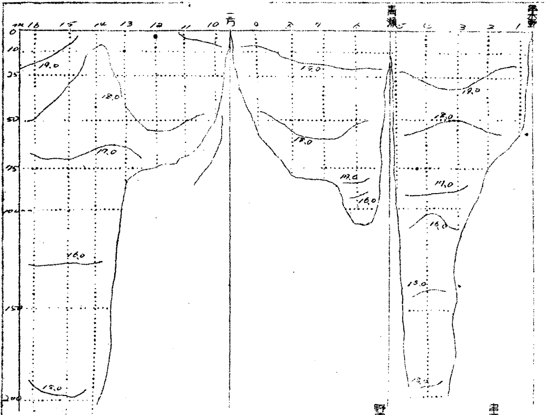
水温鉛直断面分布図 ( ^{\circ}\text{C} ) (五月)
