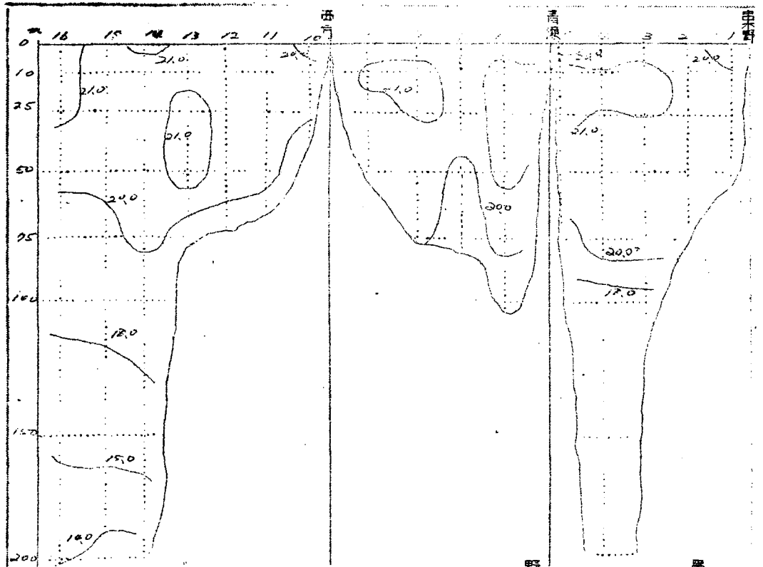
水温鉛直断面分布図 〔℃〕(十百)
