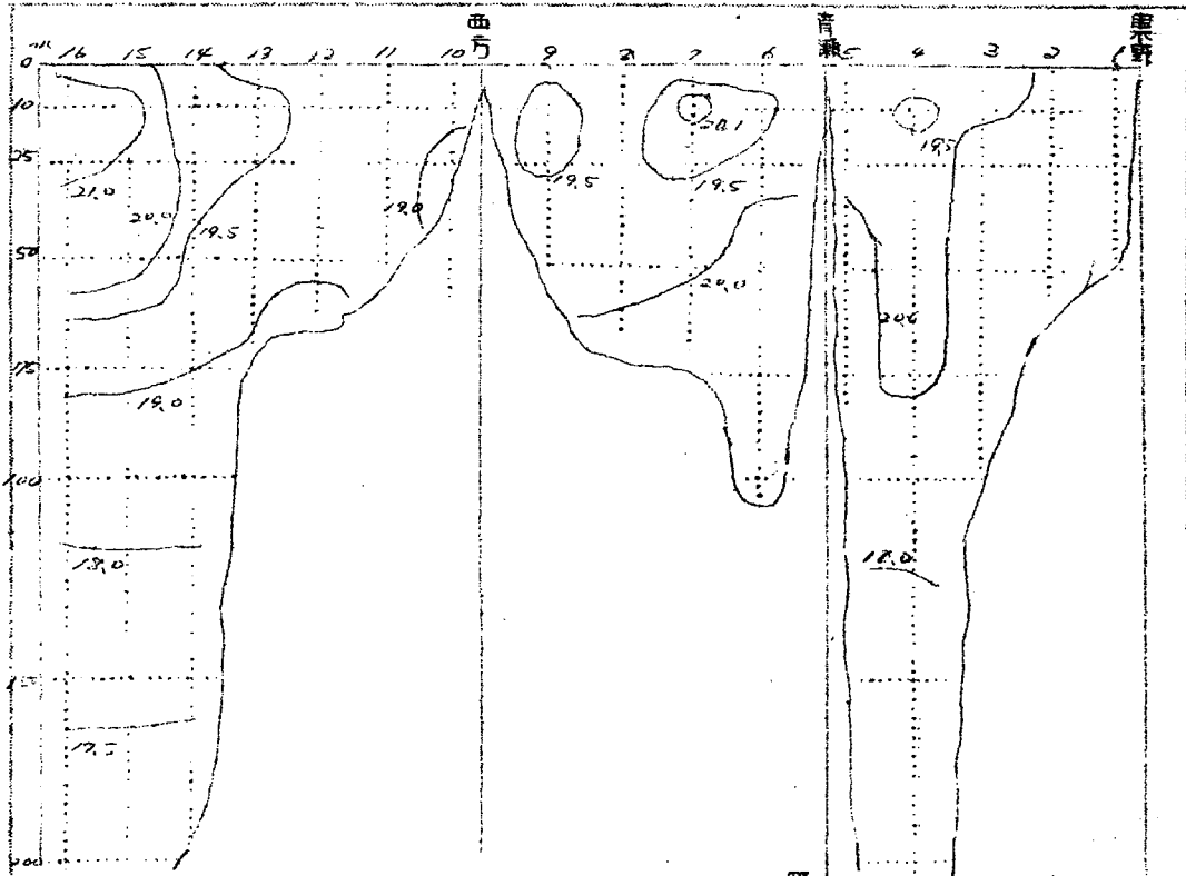
水温鉛直断面分布図
