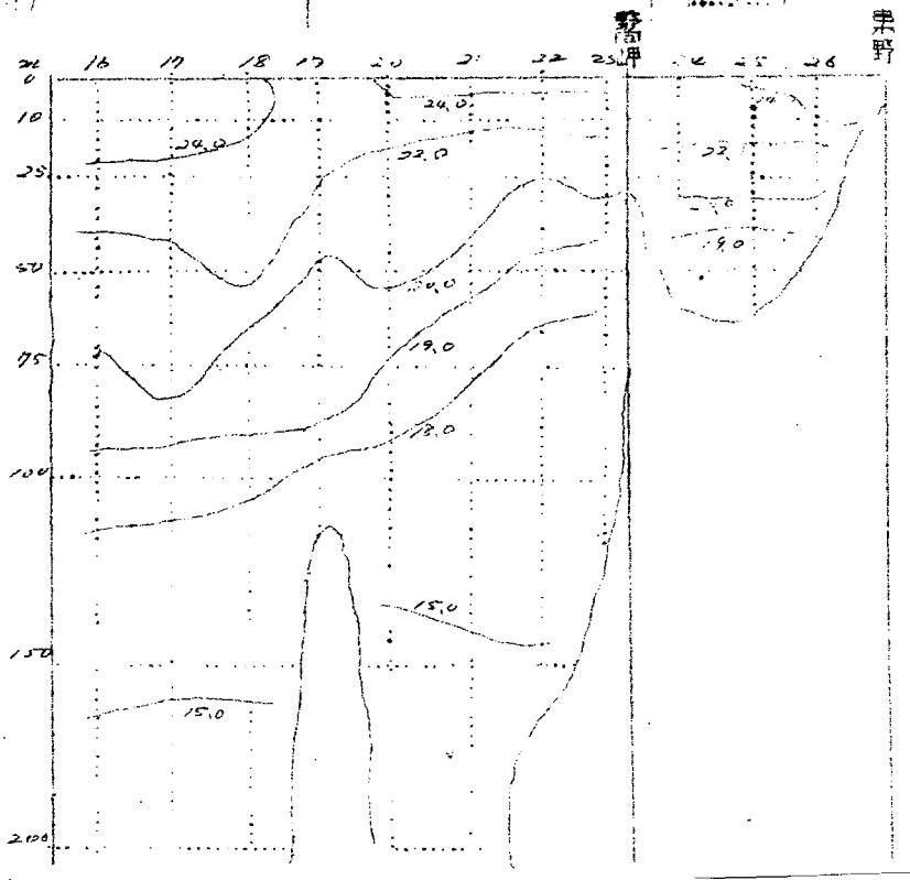
水温鉛直断面分布図 (°C) (七月)
