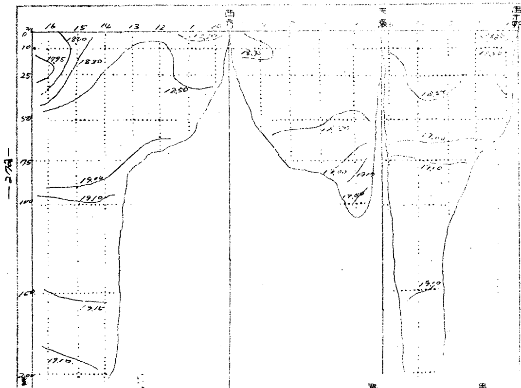
塩分飽和断面分布図 (塩素量) (一九日)
