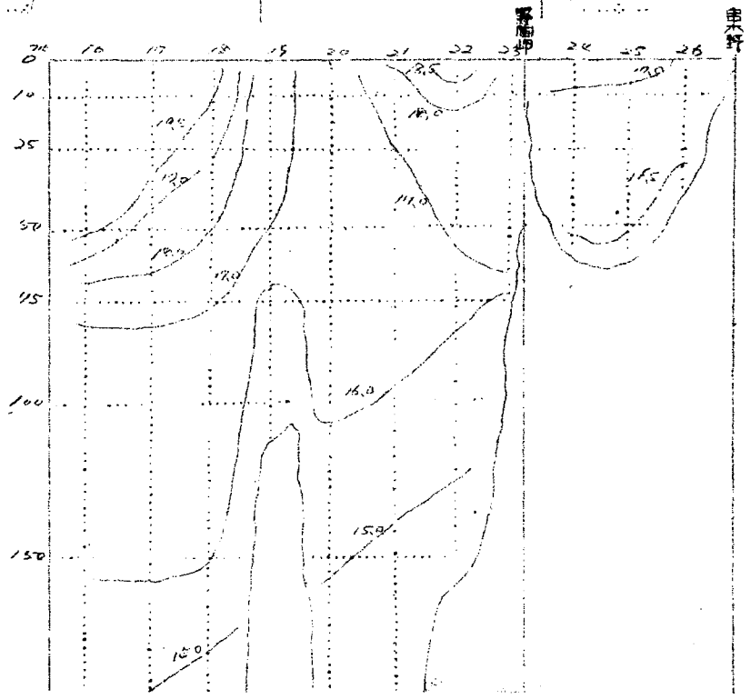
水温鉛直断面分布図 ( ^{\circ}\text{C} ) [三月]
