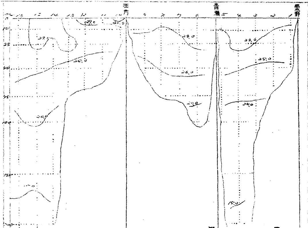
水温鉛直断面分布図 (°C) (八月)
