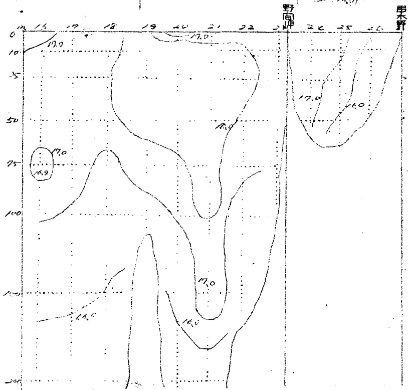
水温鉛直断面分布図 〔°C〕（二月）
