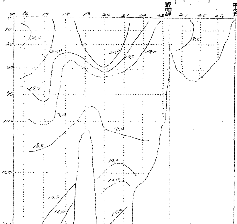
水温鉛直断面分布図
