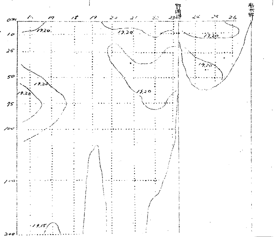
極分鉛直断面分布図 (一) 極素(%) (二) 日
