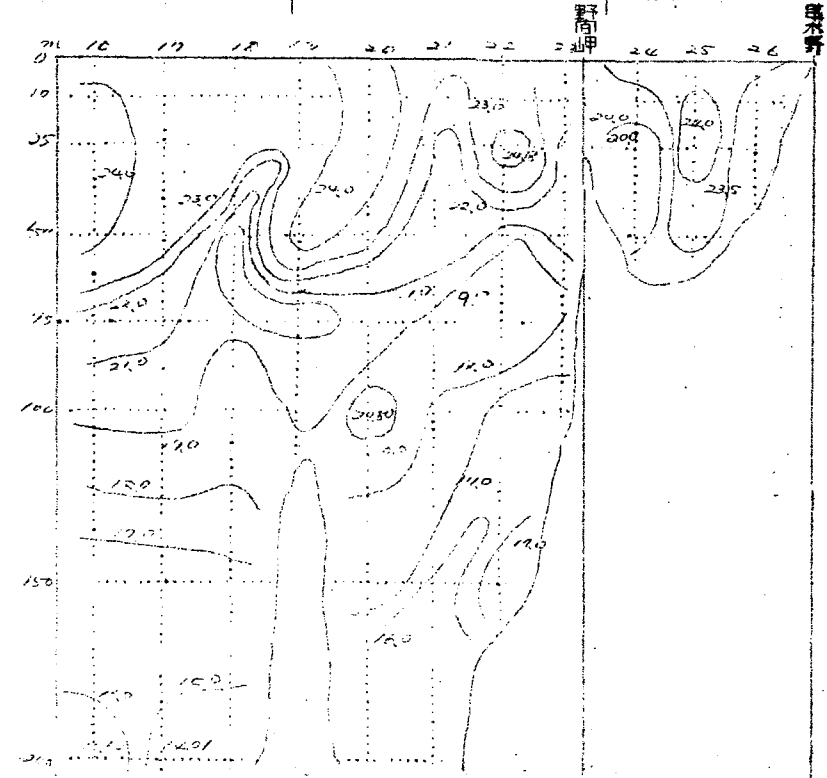
水温鉛直断面分布圖 〔C〕十一月
