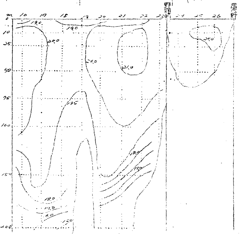
水温鉛直断面分布図 〔℃〕(二月)
