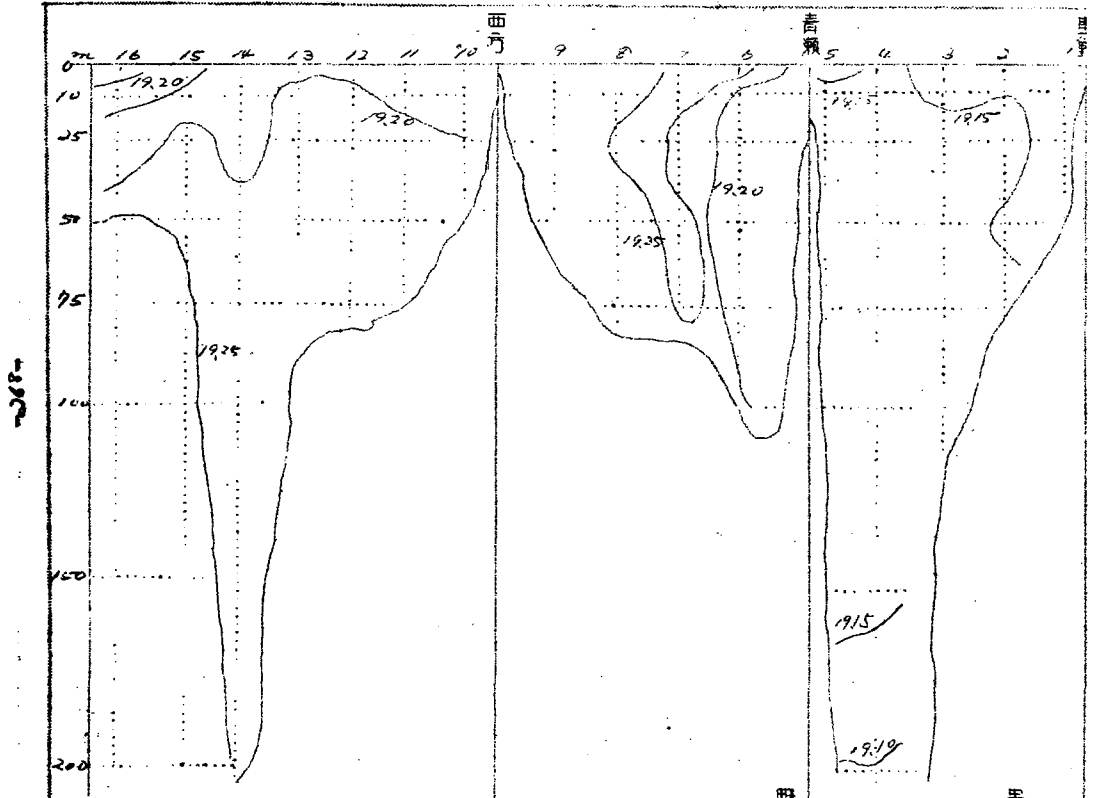
磁分鉛直断面分布図 (塩素濃度%) (五百分)
