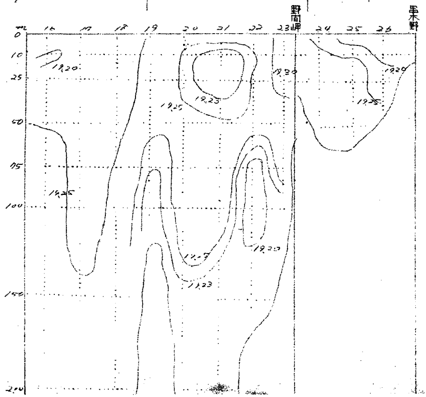
磁分鉛直断面分布図 (塩素濃度%) (五百分)
