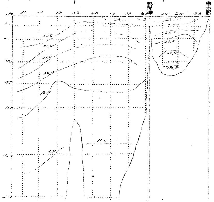
木温鉛直断面分布圖 ( ^{\circ}\text{C} ) (一二月)
