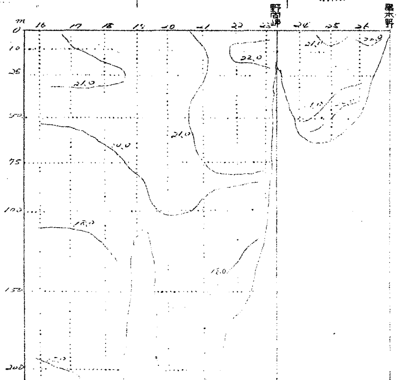
水温鉛直断面分布図 〔℃〕(十百)
