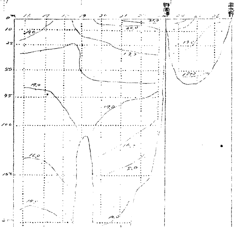
水温鉛直断面分布図 ( ^{\circ}\text{C} ) (五月)
