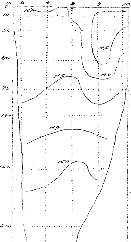
水温鉛直断面力布図 (四月) (°C)
