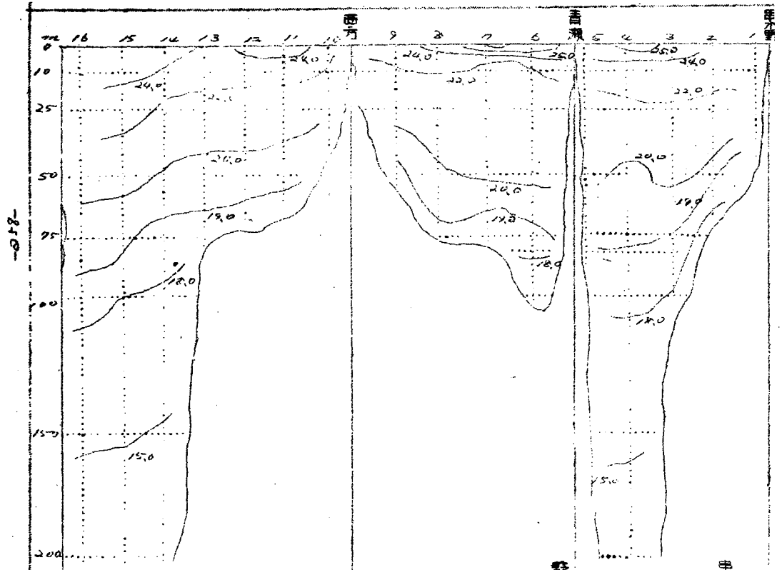
水温鉛直断面分布図 (°C) (七月)
