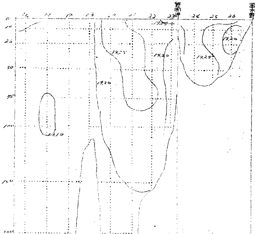
塩分飽和断面分布図(塩素量) % (二色)
