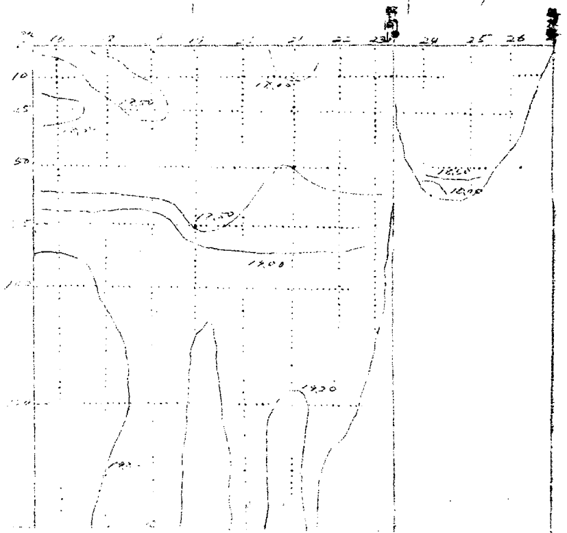
通分钻直断面分布图 (通泰堡) (八月)
