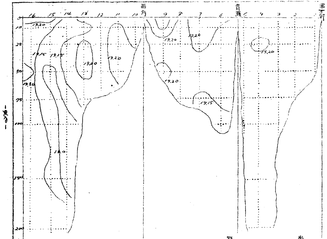
極分鉛直断面分布図 (一) 極素(%) (二) 日
