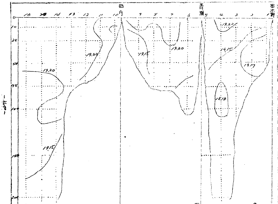
塩分鉛直断面分布図 (一) 塩素量 (%) (三月)
