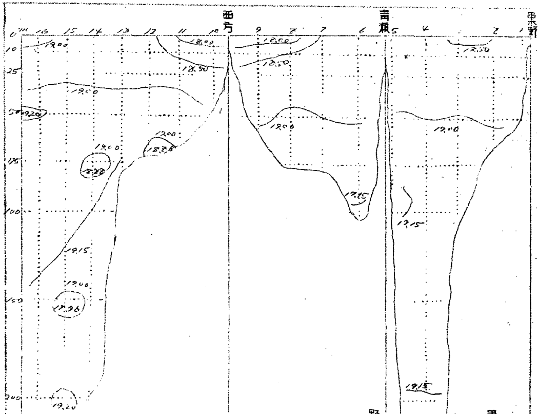
塩分鉛直断面分布図(塩分量)%(六月分)
