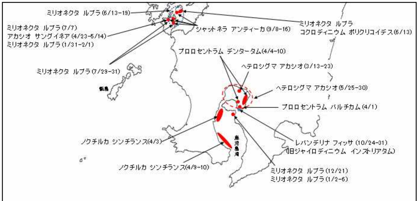
図-1 鹿児島県海域における平成28年の赤潮発生状況 (平成29年3月31日現在)
