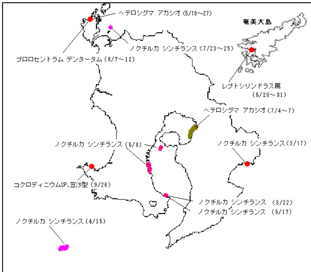
図-1 鹿児島県海域における平成24年度赤潮発生状況 (平成25年3月31日現在)
